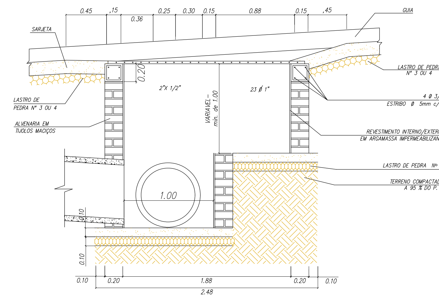
DETALHE BOCA DE LOBO Escala 1/25
