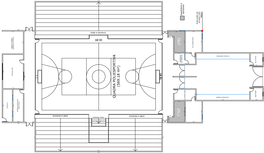
PLANTA GINÁSIO POLIESPORTIVO esc. 1/125
